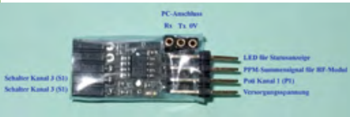
Das elektronische Kernstück des im Text erwähnten speziellen Fesselflugsenders.
